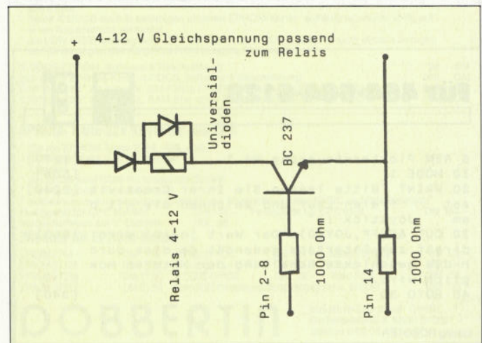
Abbildung 1: Schaltbild der Transistor-Verstärkerschaltung mit Relais
