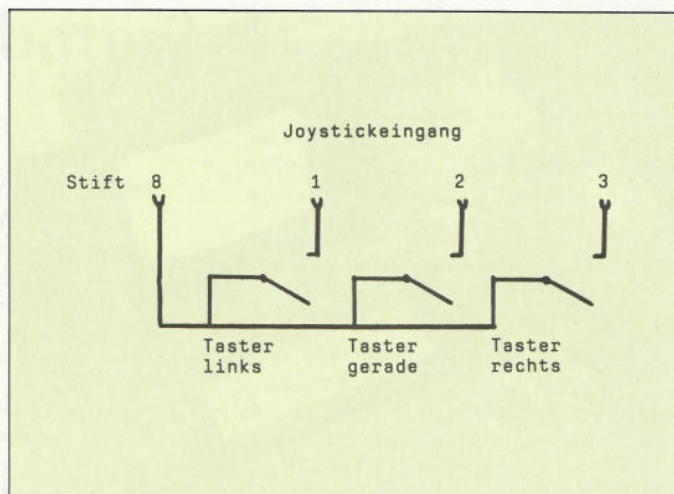
Abbildung 3: Verdrahtung der Positionstaster mit dem Joystick-Eingang
