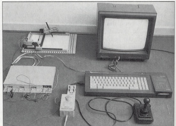
Bild 2: Der verdrahtete Gesamtaufbau des Plotters
